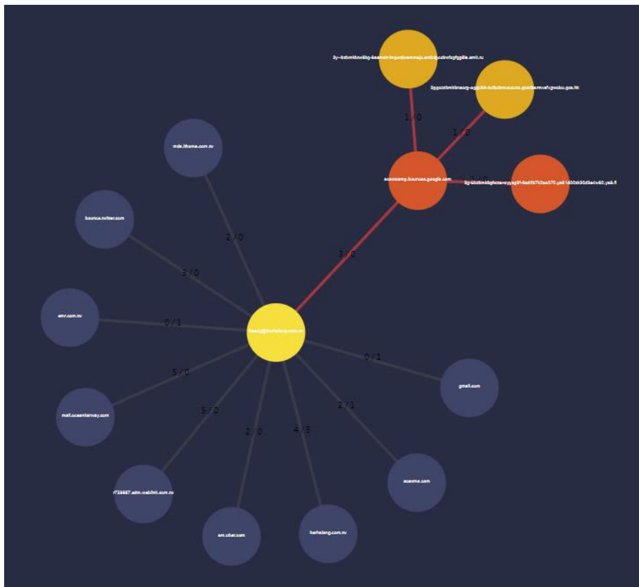
圖 2-18-2、郵件通聯圖
