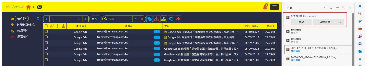
圖 2-4-6、儲存壓縮檔
