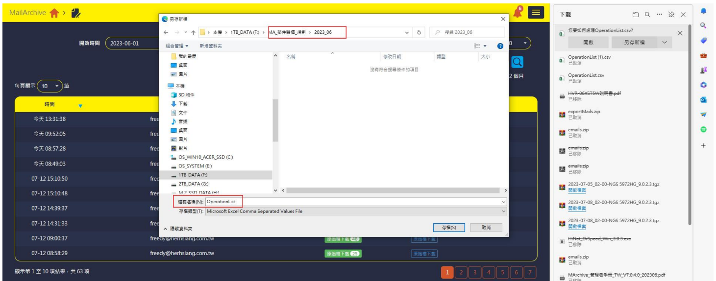
圖 2-10-6、目錄存檔
