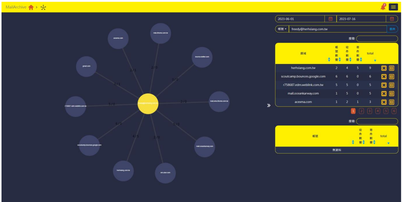
圖 2-18-1、郵件通聯圖
