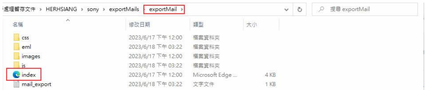
圖 2-2-19、執行 index.html
