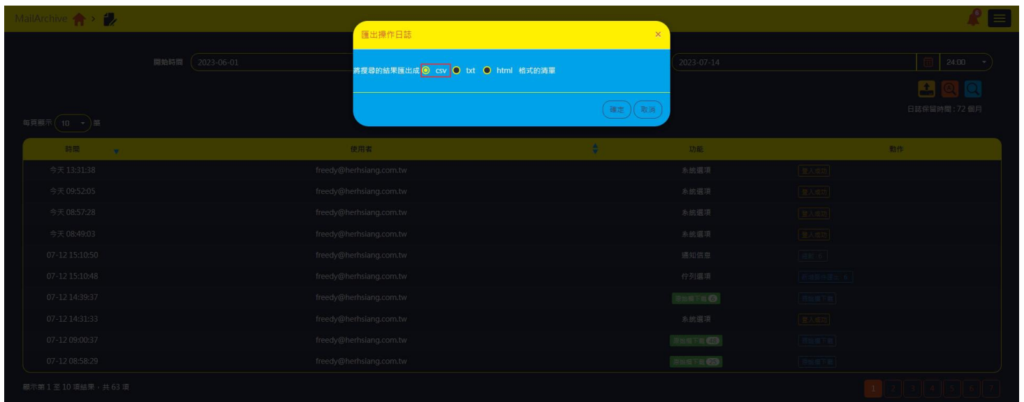
圖 2-10-4、匯出檔案
