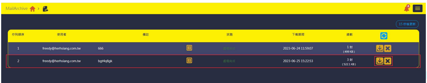
圖 2-2-15、匯出檔案
