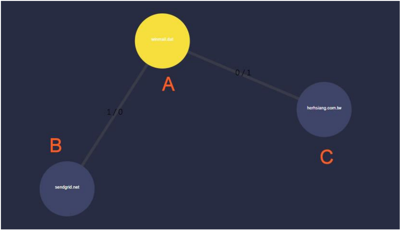
圖 2-18-4、檔案履歷
