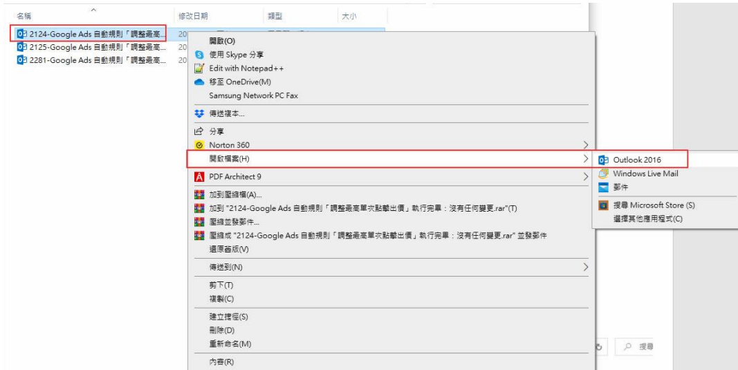
圖 2-2-11、選收信軟體
