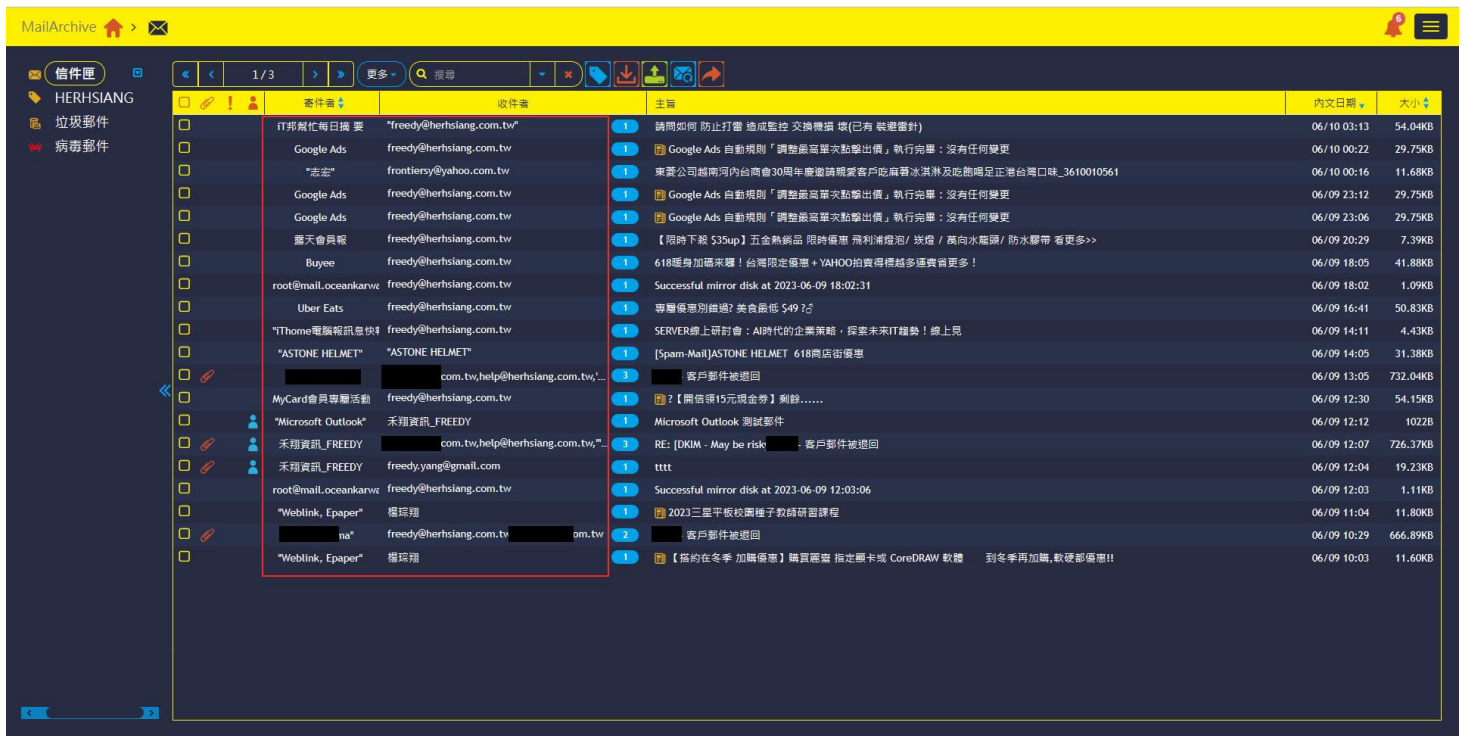
圖 2-11-11、關聯式停用
