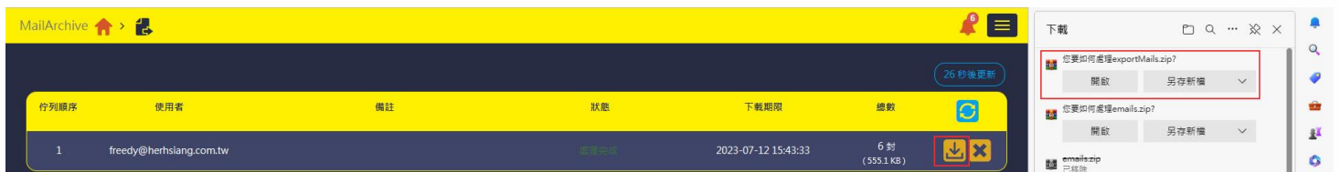
圖 2-4-9、儲存壓縮檔
