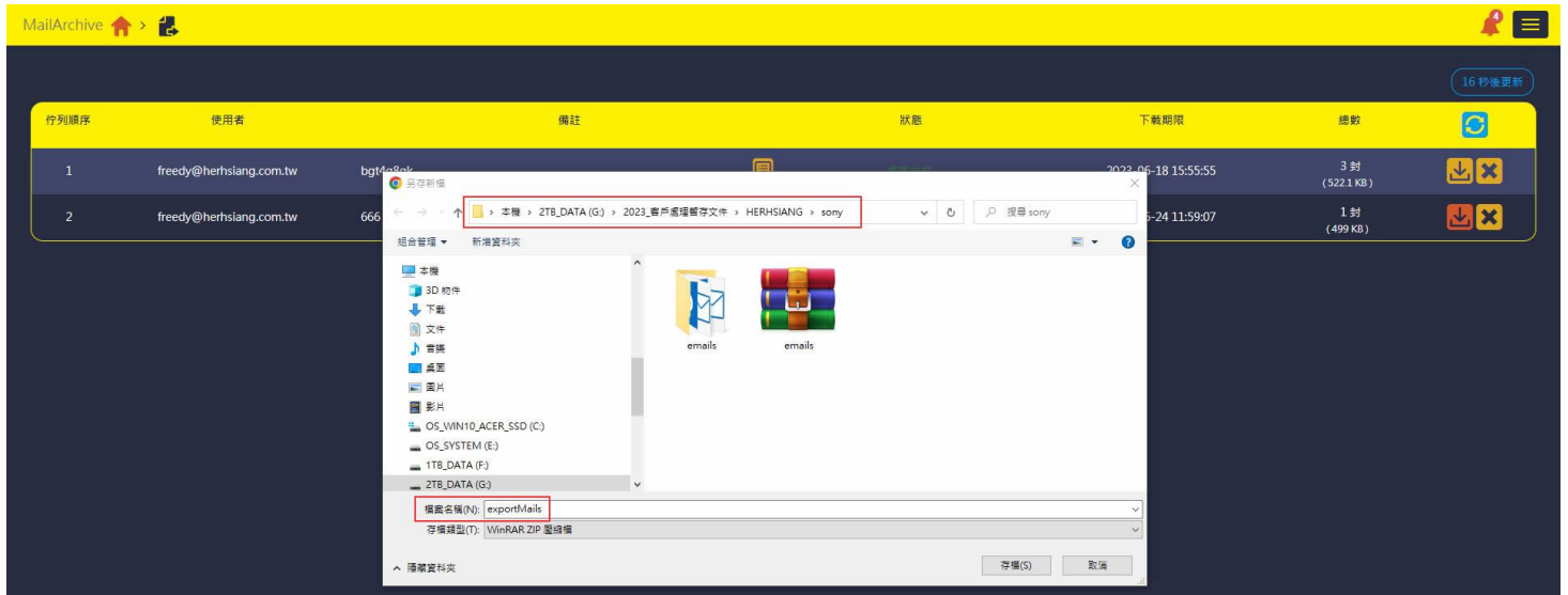
圖 2-2-16、檔案路徑
