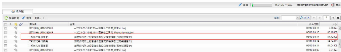
圖 2-2-26-1、郵件確認 ( 1 )
