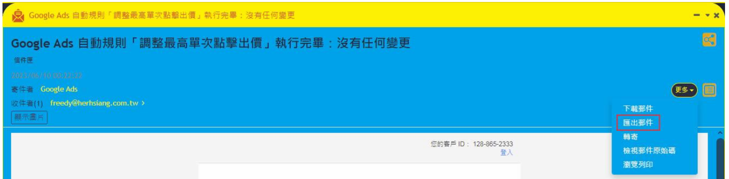
圖 2-1-2-2-3、匯出郵件
