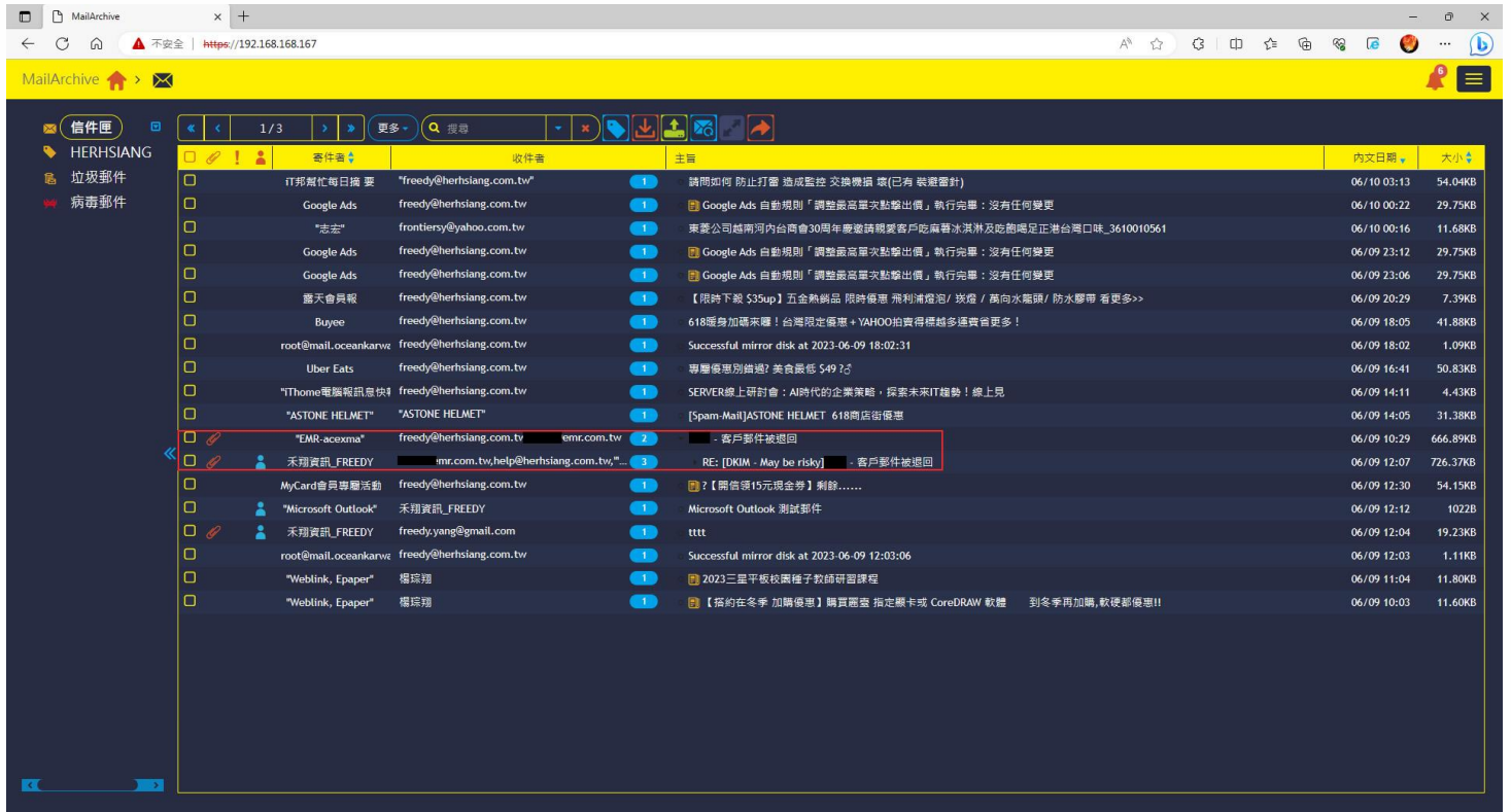
圖 2-11-12、關聯式啟用
