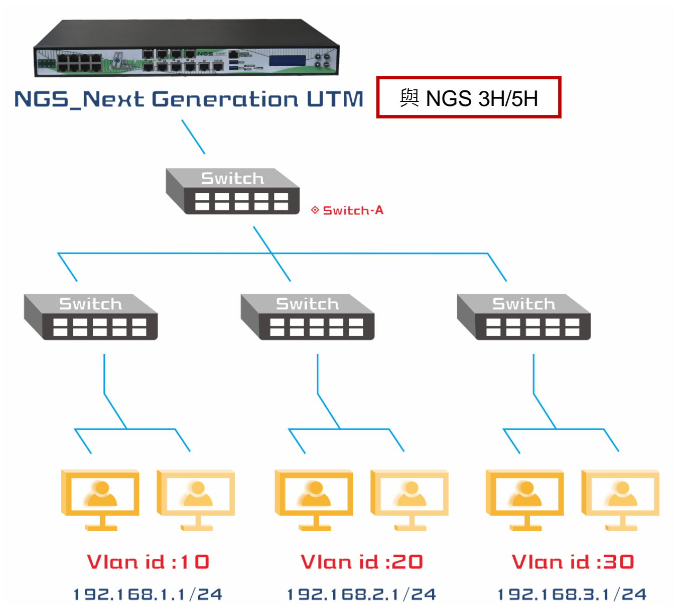
圖 3-10 VLAN 範例 (NGS 3H/5H 適用)
