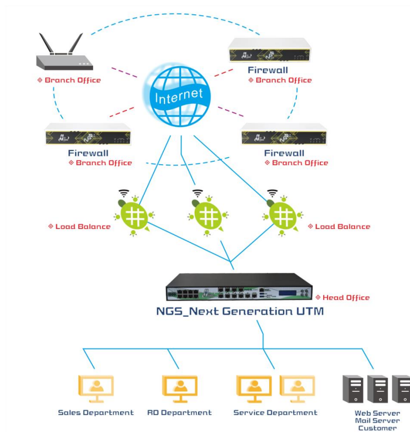
圖 1-3 建議的網路配置圖
