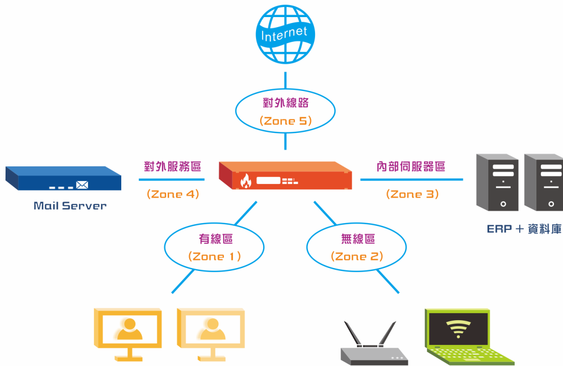
圖 4-22 管制範例網路架構圖
