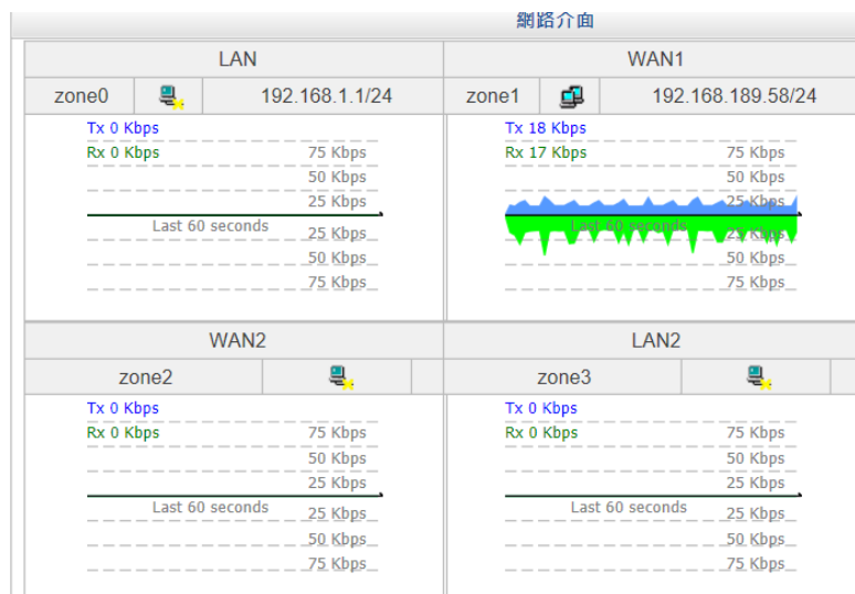
圖 1-8 NGS 3H/5H 網路介面即時流量
