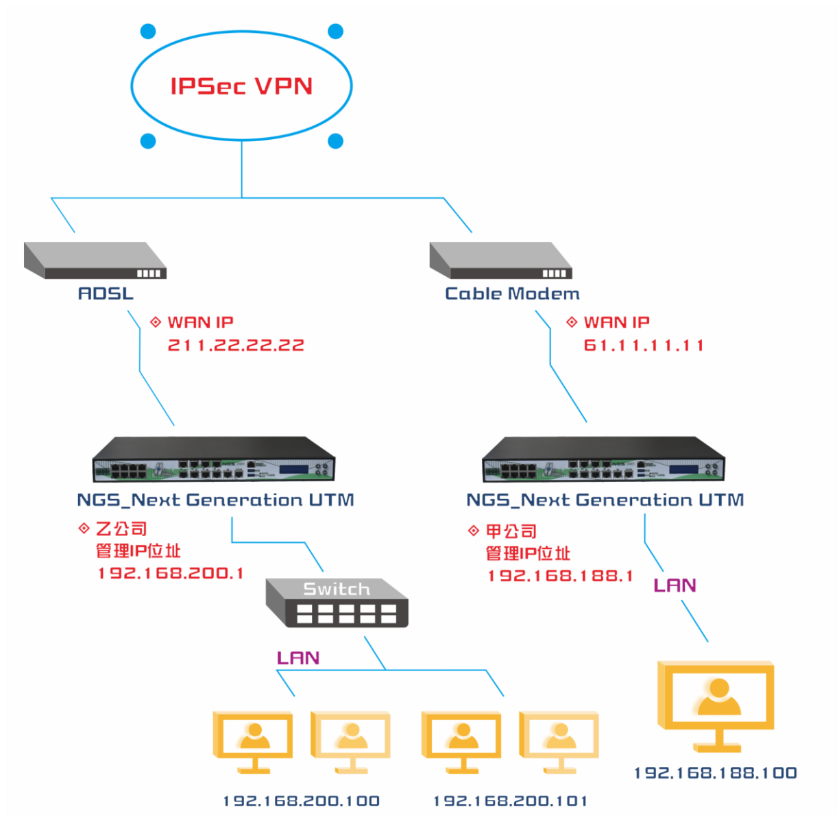
圖 12-6 IPSec VPN 連線之架設環境
